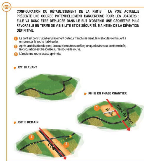
Synoptique de la configuration du rétablissement.
