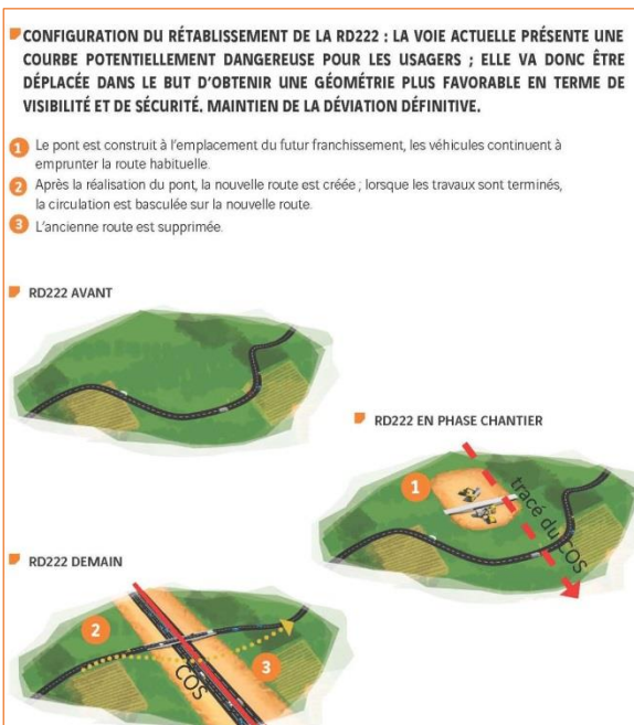
Synoptique de la configuration du rétablissement de la RD222
